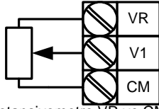
Potansiyometre VR ve CM terminallerine bağlandığında
